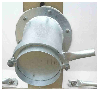
Hublot sur cône et première rehausse
